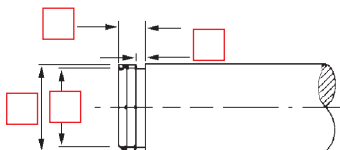
Type 4 : Embout avec gorge pour circlip
