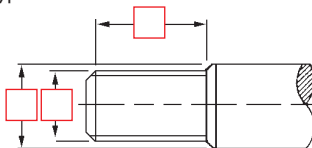
Type 2 : Embout fileté
