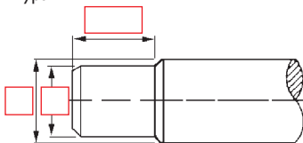
Type 2 : Embout fileté
